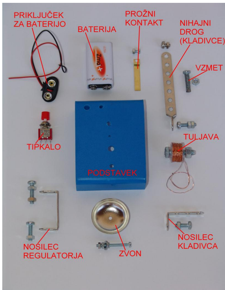
Sestavni deli zvonca brnača
