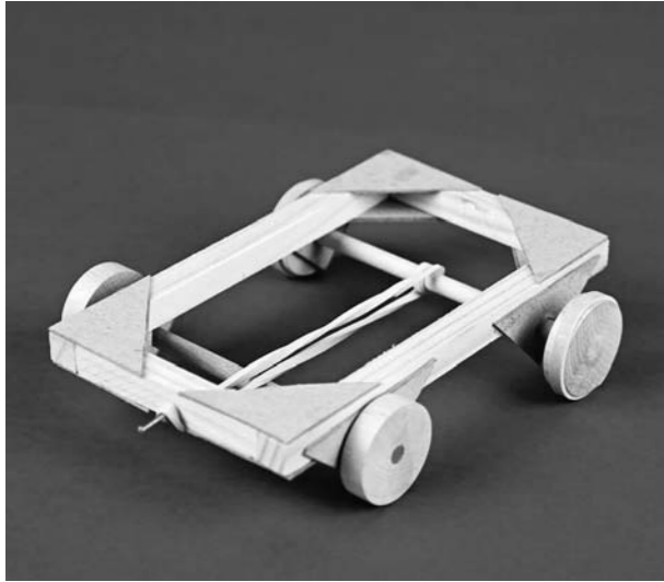
voziček s pogonom na gumo
